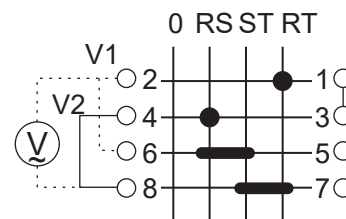
3 \phi 3 Wire
